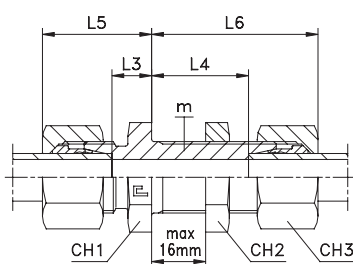
Type: 1036.. B3 Ring
