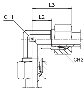
Type: 1038.. B3 Ring
