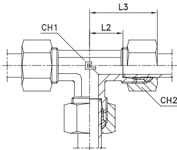
Type: 1039.. B3 Ring
